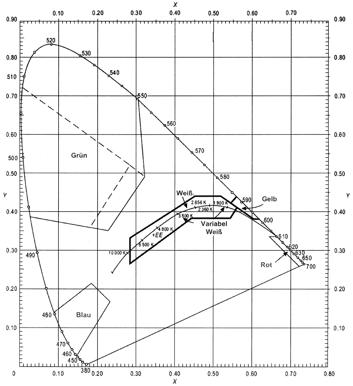
Abbildung 5-13. Farbdiagramm Randfeuer
