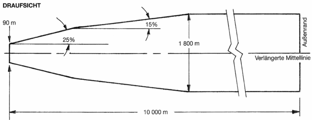
PROFIL: 3°- Anflug
