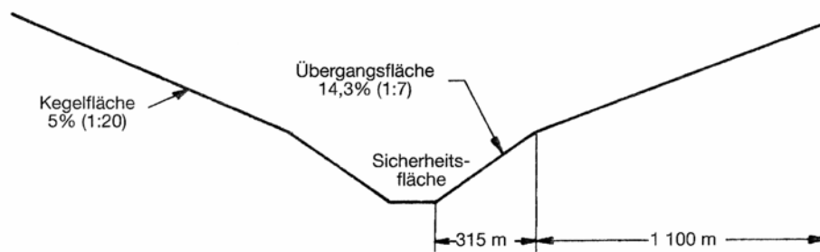
Alternative, wenn keine innere Horizontalfläche vorhanden ist
