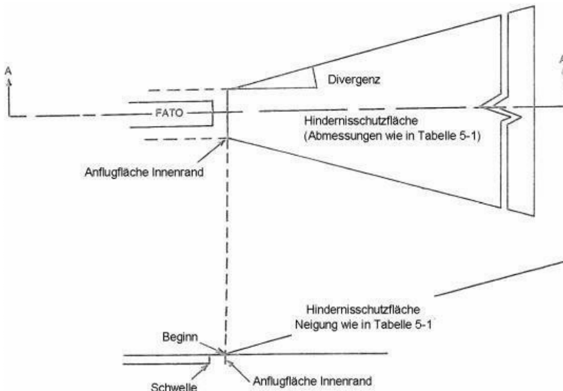
Abbildung 5-12. Hindernisschutzfläche für Gleitwinkelbefehrerungen
