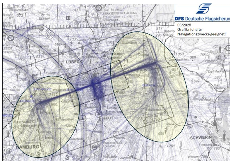
Graphik 2: IFR-Anflugströme nach Lübeck und „Awareness-Bereiche“
